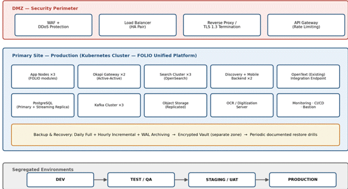
الشكل 3: معمارية النشر — الإنتاج والبيئات المنفصلة
